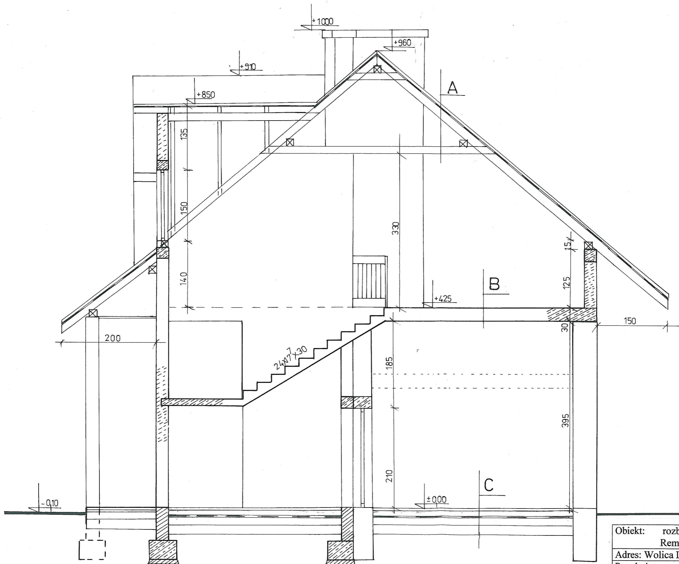
PRZEKRÓJ H 1:50
