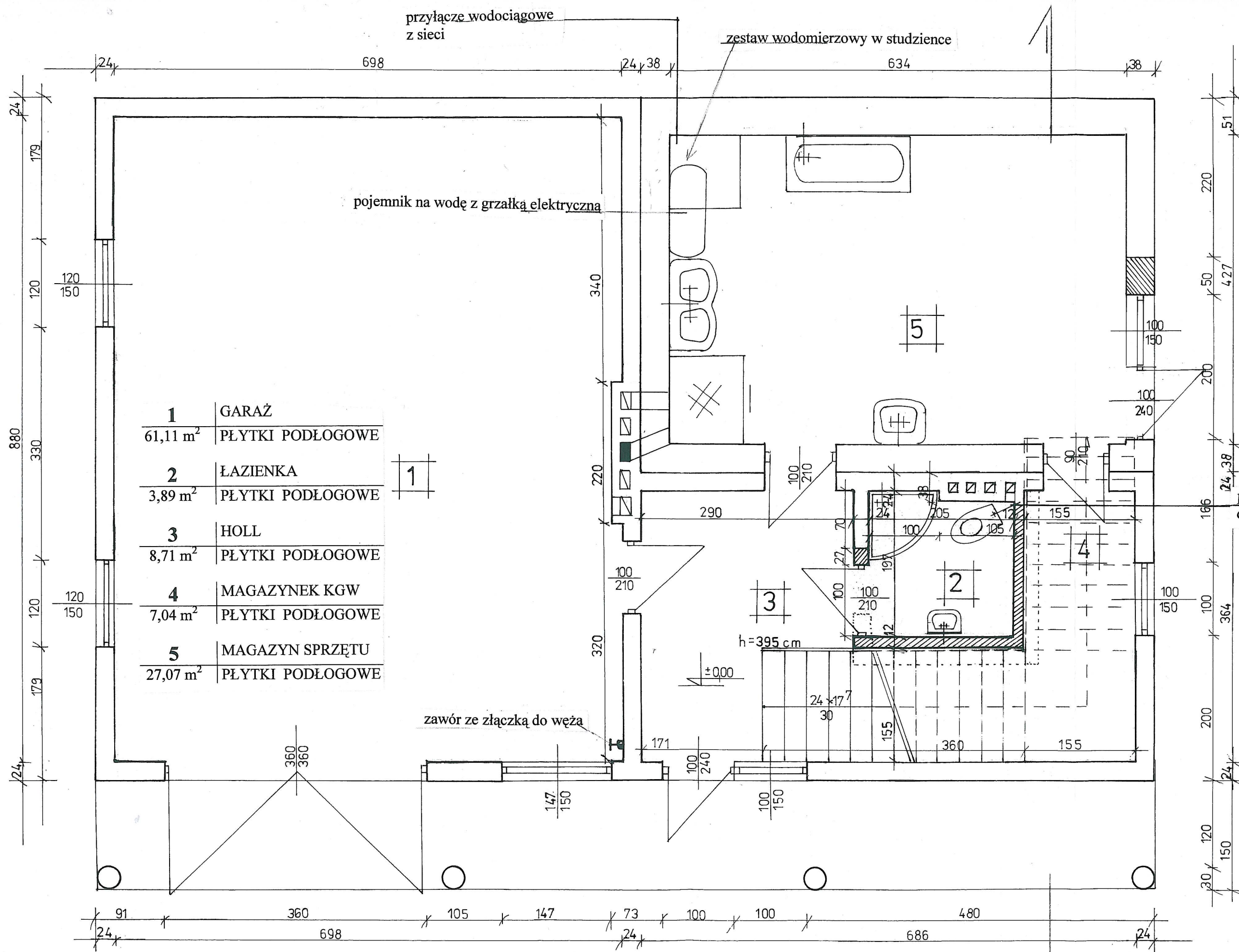
RZUT PARTERU 1:50
