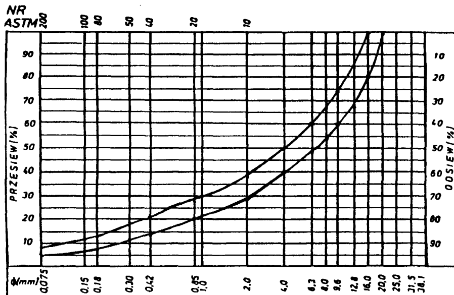
Rys. 4. Krzywe graniczne uziarnienia mieszanki mineralnej 0÷20 mm do warstwy ścieralnej z betonu
